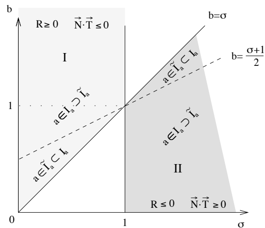
FIG. I-39 – Intervalles possibles pour a pour que les surfaces (I.B-1) soient semi-perméables ( \vec{I}_a \equiv \hat{I}_a ).
