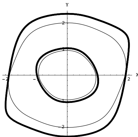
FIG. II-10 – Les deux cycles limites du système (II.2-3) en trait gras et leurs approximations algébriques en trait fin H_6(x, y) = k_{1,6}^* et H_6(x, y) = k_{2,6}^*
