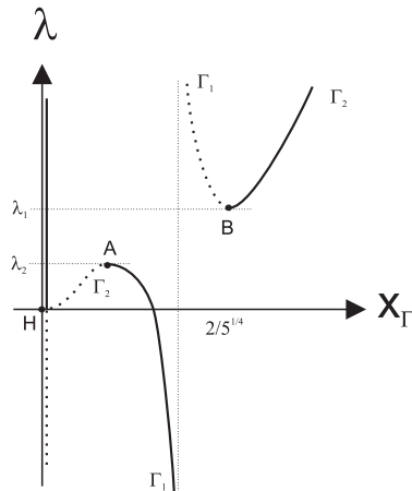
FIG. IV-13 – Diagramme de bifurcation des points d'équilibre et des cycles limites du système (IV.2-2). La droite x = 0 représente le point d'équilibre à l'origine. Les courbes en pointillés indiquent le caractère instable de la solution asymptotique (cycle limite ou point d'équilibre), alors que les courbes en traits pleins indiquent la stabilité.
