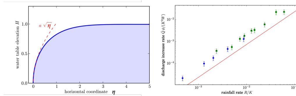
FIGURE 19 – Gauche : résolution de l'équation du régime de tempête ( storm flow ), image de Guérin et al. A droite : débit de sortie en fonction du tau de pluie R pour deux expériences 4 mm glass beads (blue dots) and 1 mm glass beads (green squares). La ligne rouge est le régime asymptotique q(0, t) \propto R^{3/2} .
