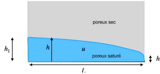
FIGURE 15 – Exemple de cas d'écoulement en couche mince dans un milieu poreux : deux retenues d'eau de hauteur h_1 et h_2 séparés par une distance L de percolation,
