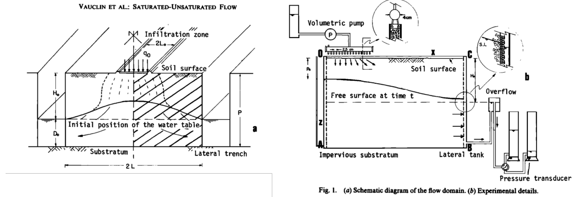
FIGURE 23 – Expérience de Vauclin et al, 1979, Water Resources Research
