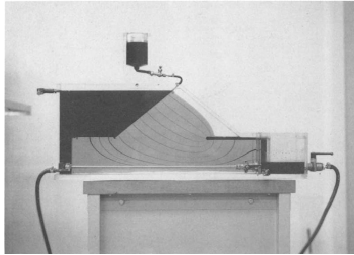
FIGURE 10 – Exemple d'expérience de la boratoire montrant l'écoulement d'infiltration dans un massif poreux, (barrage en terre). Cette visualisation a été obtenue à l'aide d'une cuve d'Hele-Shaw verticale, et montre clairement la forme de la surface libre et les lignes de courant de l'écoulement potentiel. (Photographie réalisée au laboratoire d'hydrodynamique de l'E.N.S.T.A). Photo du livre de Darrozès & François Cours Mécanique des Fluides de l'ENSTA
