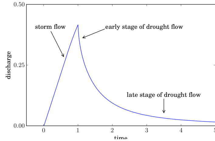
FIGURE 20 – Réponse q(x=0, t) d'un aquifère à un créneau de pluie R(t < .25) = 1 et R(t > .25) = 0 (issu de Guérin [5]).
