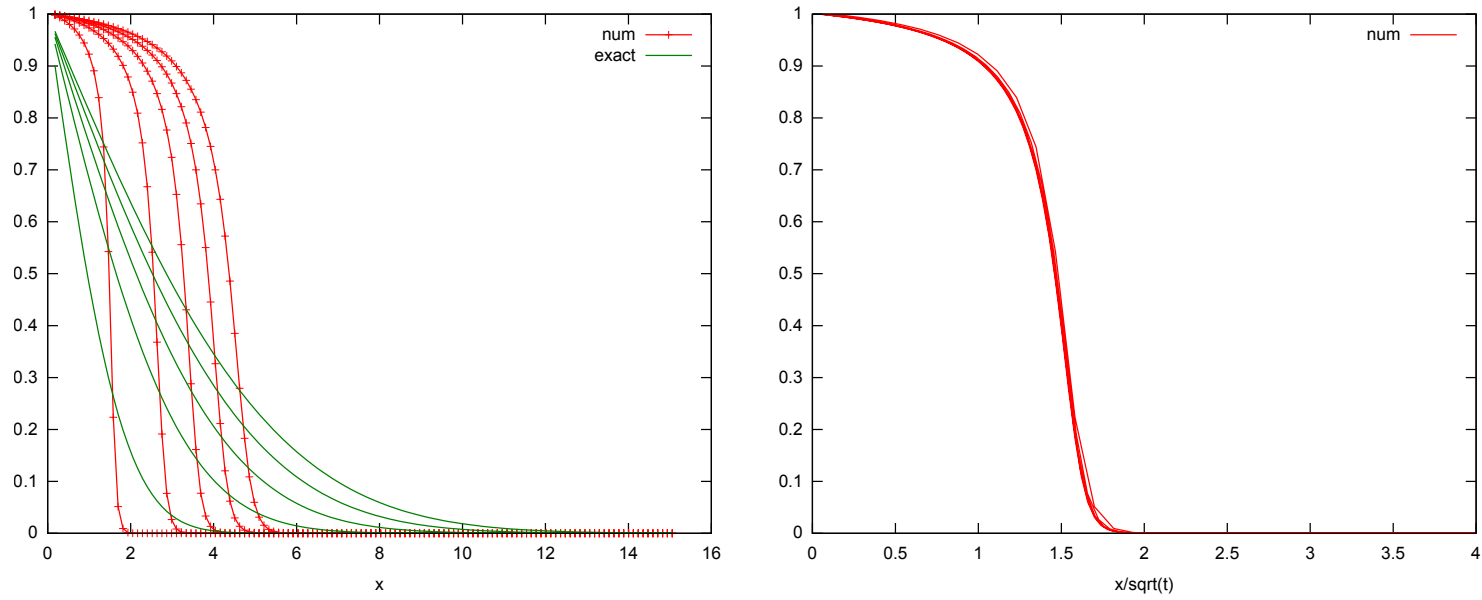
FIGURE 21 – Résolution de l'équation d'imbibition de Richards, avec D = (0.05/(1.05 - \theta))^2 en rouge. En vert le cas à coefficient D constant de la diffusion classique. A gauche, avancée du front en fonction du temps, à droite superposition de la solution semblable x/\sqrt{t} .
