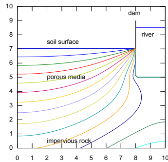
FIGURE 8 – Exemple de cas d'écoulement sous un barrage, tout est mouillé, calcul Basilisk , gauche et centre iso pression. Droite charge hydraulique H = h + z .
