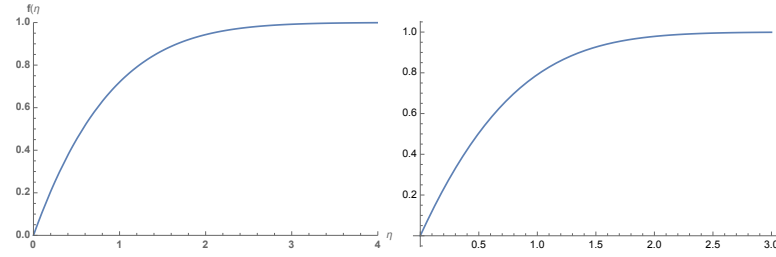
FIGURE 17 – Solution autosemblable, gauche \text{erf}(\eta/2) = \frac{2}{\sqrt{\pi}} \int_0^{\eta/2} e^{-\xi^2} d\xi de l'équation linéarisée dans le cas d'une sortie de quasi même niveau que l'aquifère initial, droite solution semblable linéarisée du cas avec pluie solution -\sqrt{\frac{\pi}{2}} \eta \text{erf}\left(\frac{\eta}{\sqrt{2}}\right) - e^{-\frac{\eta^2}{2}} + \sqrt{\frac{\pi}{2}} \eta + 1
