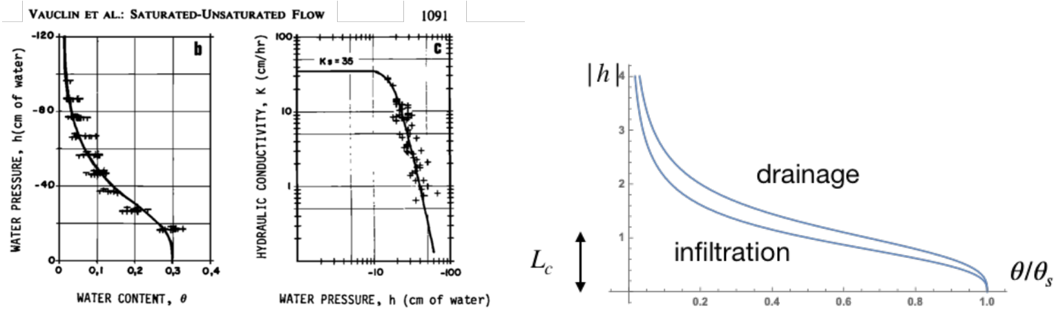
FIGURE 12 – \theta(h) et K(h) pour du sable fin de rivière tamisé (expérience de Vauclin 1979 [17]). A droite, la courbe \theta(h) peut varier entre l'infiltration et le drainage.
