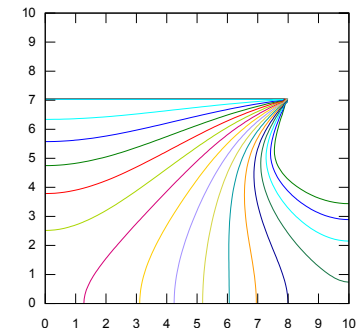
FIGURE 8 – Exemple de cas d'écoulement sous un barrage, tout est mouillé, calcul Basilisk , gauche et centre iso pression. Droite charge hydraulique H = h + z .
