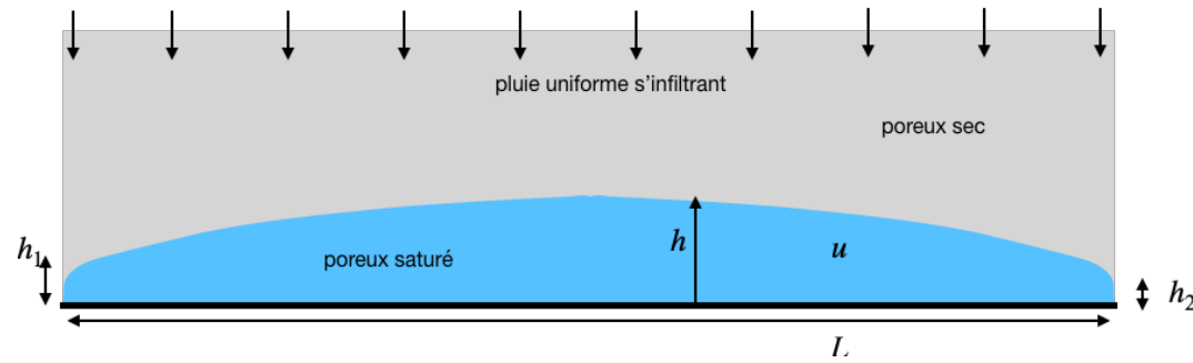
FIGURE 16 – Exemple de cas d'écoulement en couche mince dans un milieu poreux avec un terme de pluie. L' aquifère est alimenté par la pluie, il se vide à droite et à gauche.
