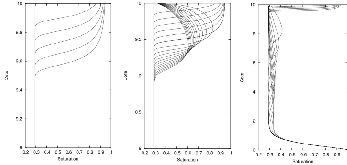
FIGURE 13 – Résolution de l'équation d'imbibition de Richards, issue de metis.upmc.fr/m2HH/Ledoux
