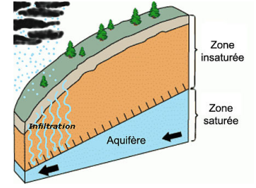
FIGURE 11 – "Nappe phréatique", une partie du cycle de l'eau, dessin sursimplifié, idéalisé de wikipedia
