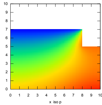
FIGURE 8 – Exemple de cas d'écoulement sous un barrage, tout est mouillé, calcul Basilisk , gauche et centre iso pression. Droite charge hydraulique H = h + z .
