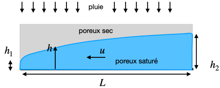
FIGURE 18 – Exemple de cas d'écoulement poreux, empilement de billes de verres entre deux plaques de verre, à droite et en bas, les billes sont retenues par une plaque de verre, à gauche par une grille. Un tube percé en eau laisse goutter une pluie. Expérience à gauche, schéma à droite.
