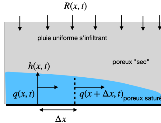
FIGURE 14 – Bilan simplifié pour établir la relation de Dupuit-Boussinesq, le poreux est supposé sec (malgré l'infiltration) et l'eau est piégée dans la nappe fine d'épaisseur h , soit q le débit circulant dans la couche d'eau. On fait un bilan sur une tranche \delta x de ce qui entre et sort.
